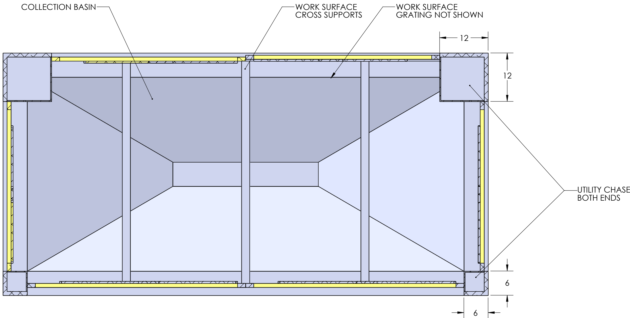
SECTION A-A
